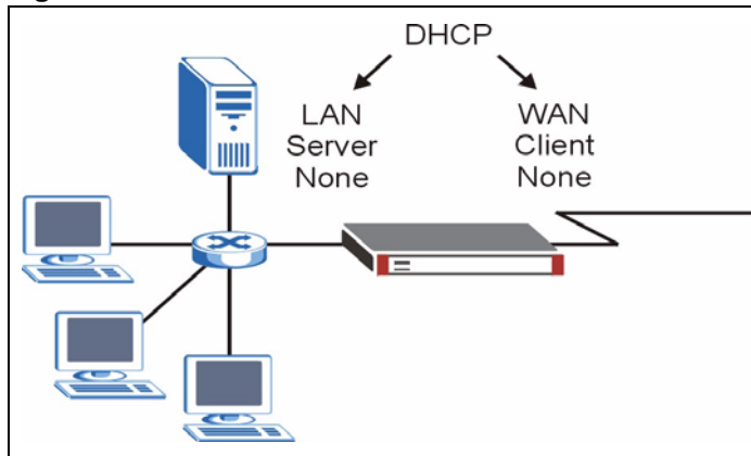
Figure 407 WAN & LAN DHCP
