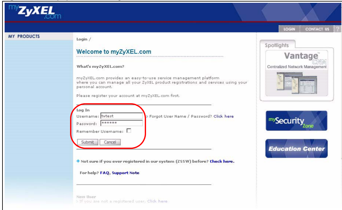
Figure 159 myZyXEL.com: Login
